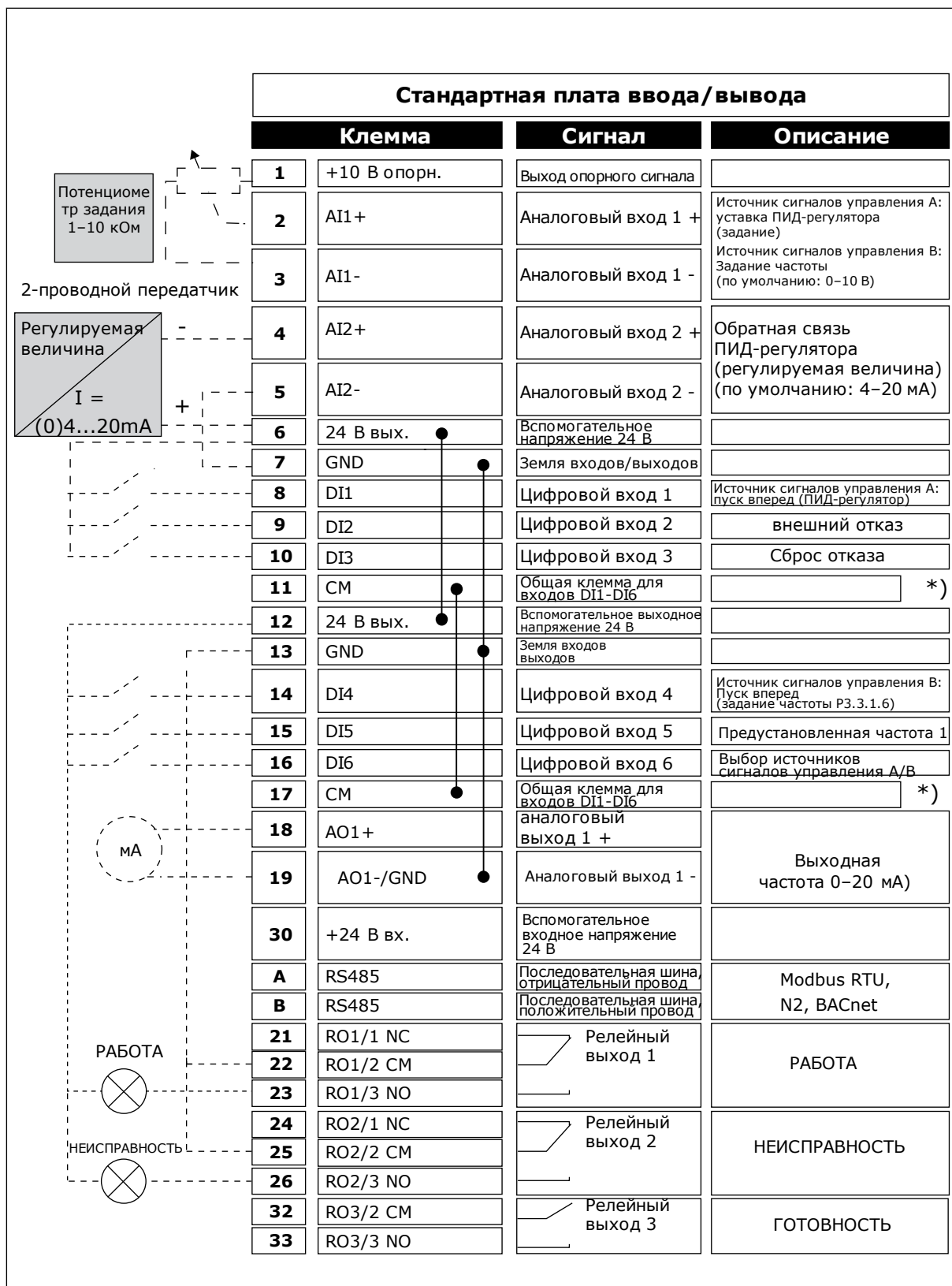
Рис. 10: Цепи управления, которые по умолчанию используются для приложения ПИД-регулирувания
