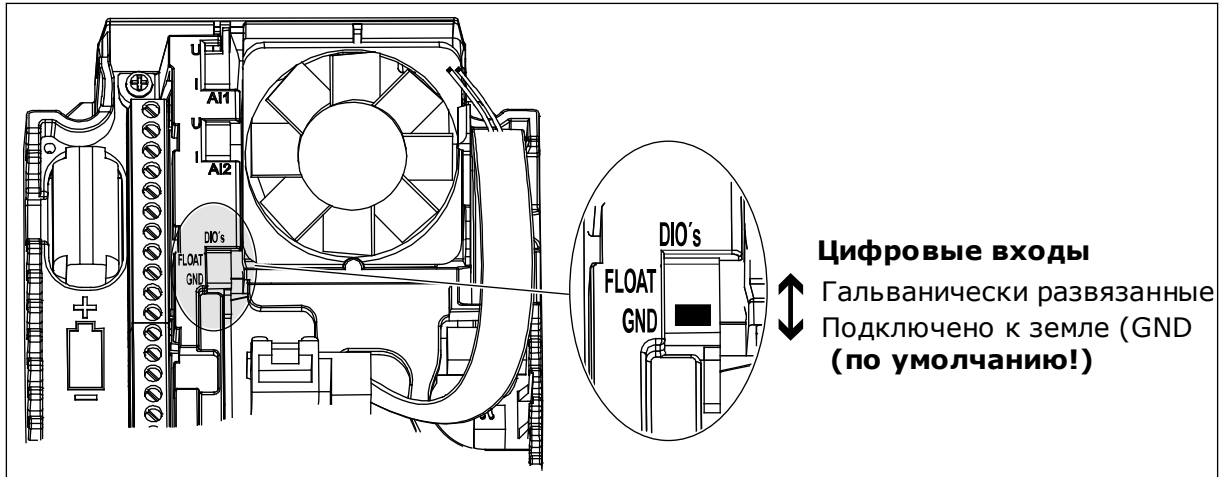
Рис. 11: DIP-переключатель
