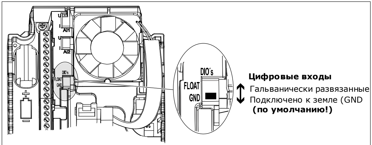
Рис. 15: DIP-переключатель
