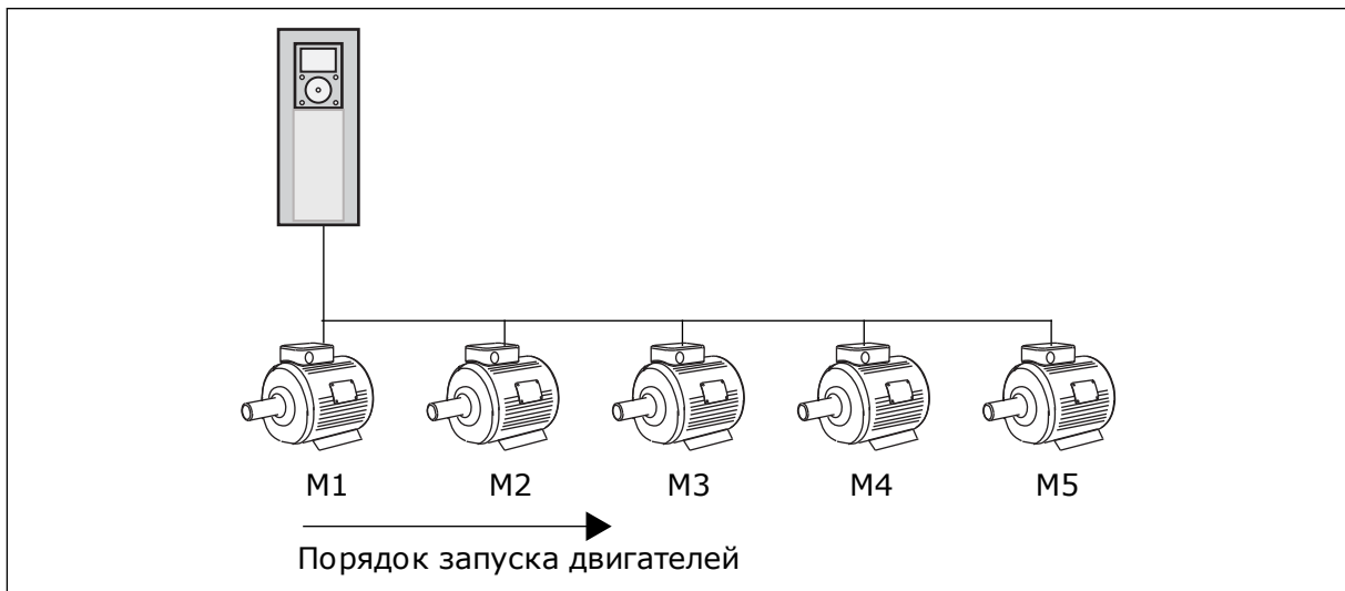
Рис. 80: Логика блокировки 1
